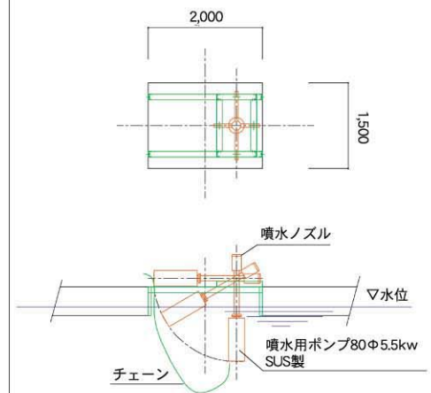
噴水ノズル、ポンプ廻り詳細図
